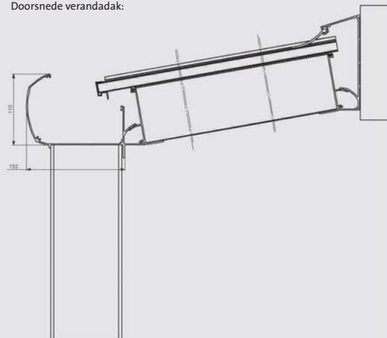
Doorsnede verandadak:
